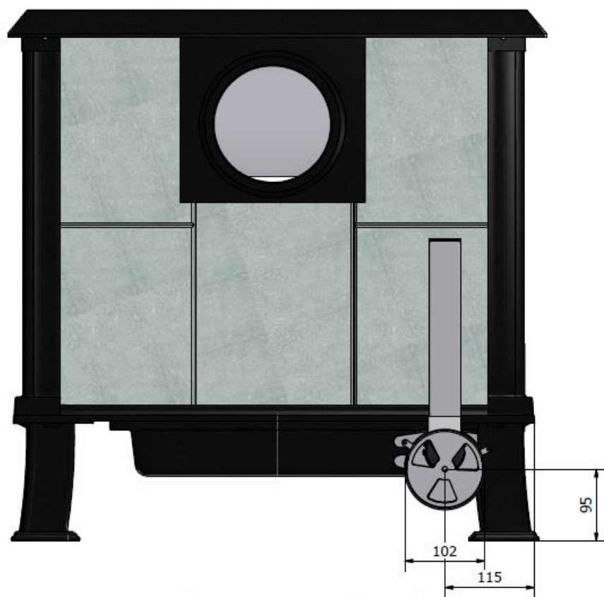
maatvoering buitenluchtset Vision (Gourmet)
